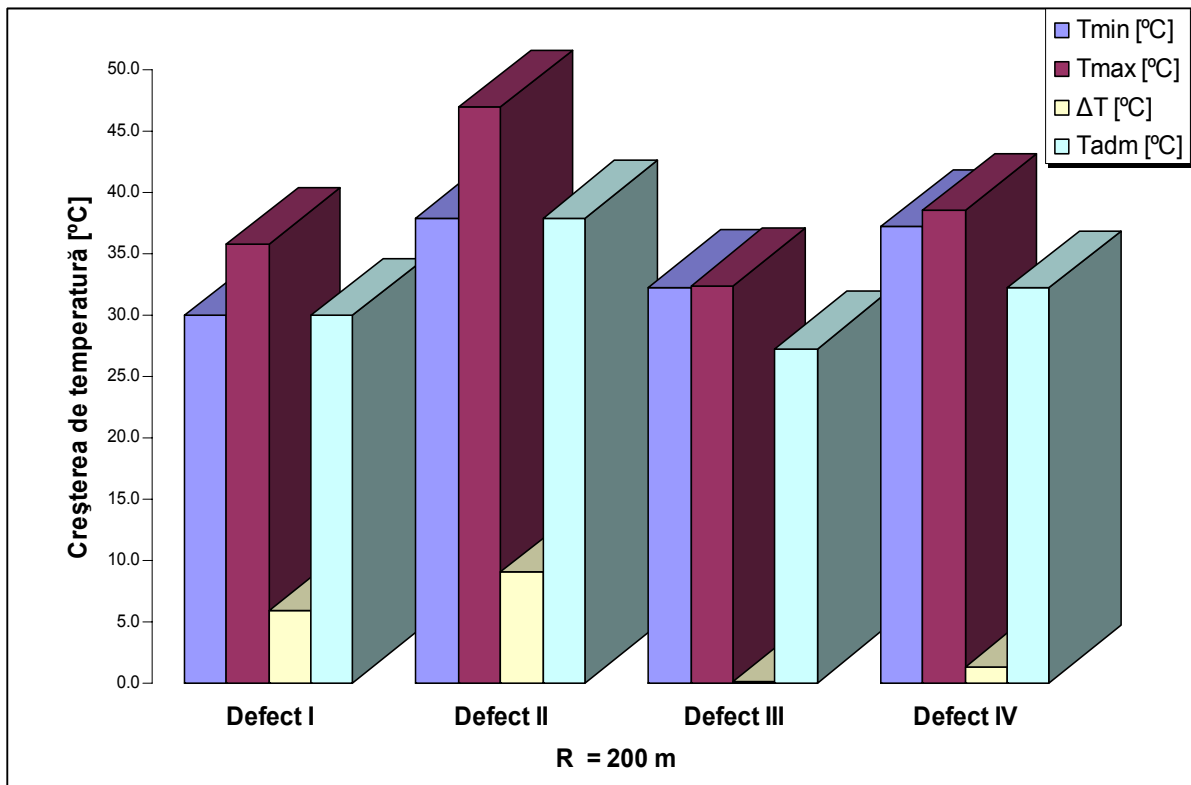
Fig. 9 Influența formei defectelor de direcție asupra șerpuirii căii, la calea în curbă cu raza R = 200 m solicitată doar la variații de temperatură
