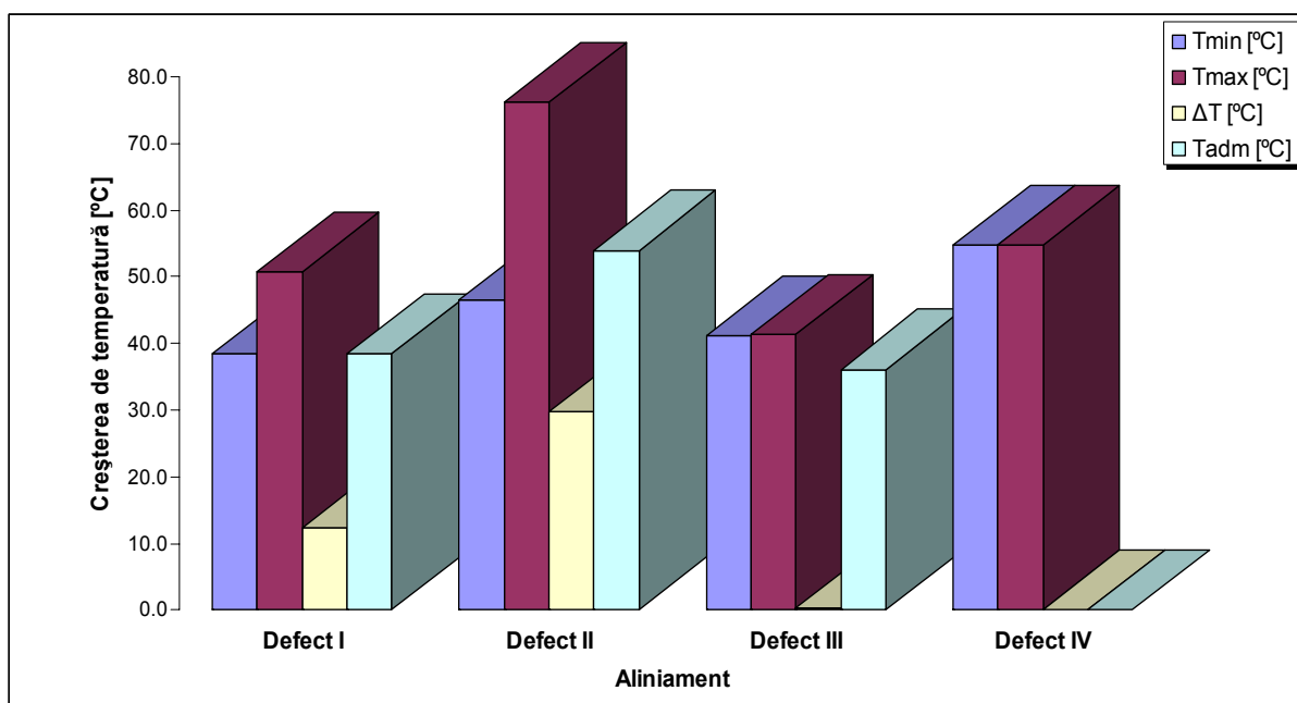
Fig. 6 Influența formei defectelor de direcție asupra șerpuirii căii, la calea în aliniament solicitată doar la variații de temperatură
