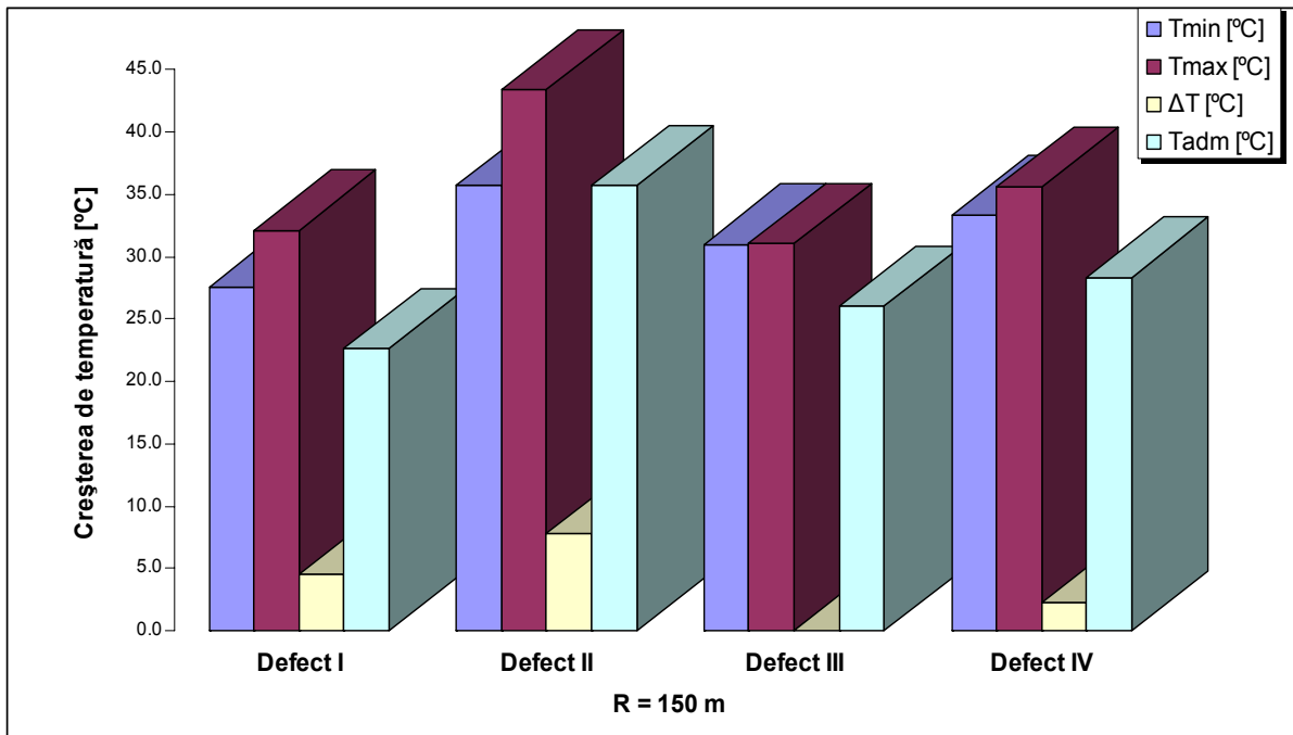
Fig. 8 Influența formei defectelor de direcție asupra șerpuirii căii, la calea în curbă cu raza R = 150 m solicitată doar la variații de temperatură
