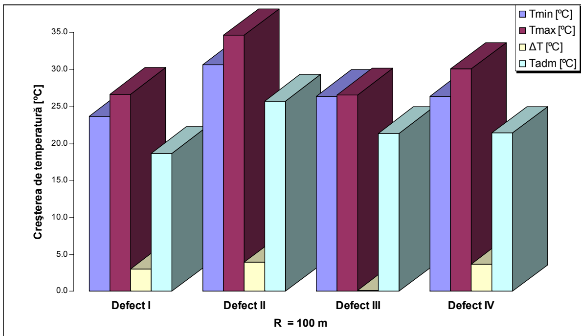
Fig. 7 Influența formei defectelor de direcție asupra șerpuirii căii, la calea în curbă cu raza R = 100 m solicitată doar la variații de temperatură
