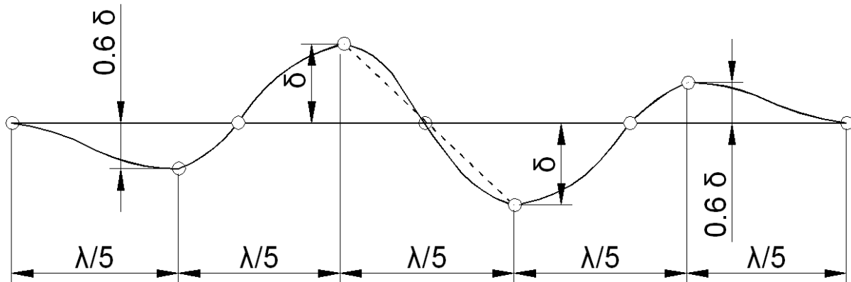
Fig. 1. Forme caracteristice ale defectelor de direcție [2]
