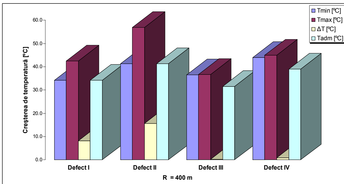
Fig. 5 Influența formei defectelor de direcție asupra șerpuirii căii, la calea în curbă cu raza R = 400 m solicitată doar la variații de temperatură
